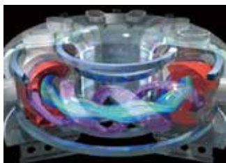
ジャイロ運動論粒子コードによる大型ヘリカル装置の炉心プラズマにおける微視的不安定性シミュレーション
